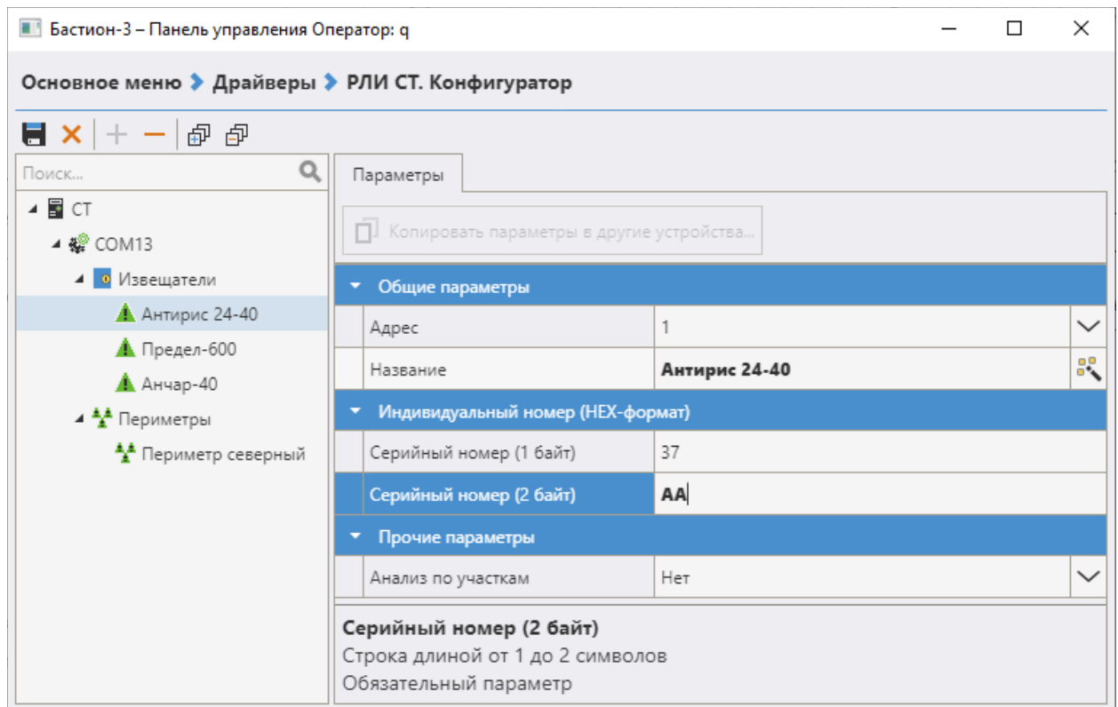
Рис. 1. Настройка извещателей
